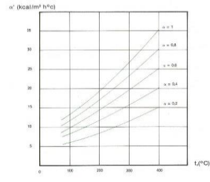
Fig. 3.5 -- Coefficiente \alpha' di dispersione termica globale, per irraggiamento e convezione naturale in aria, in funzione della temperatura della parete e della sua emissività [57]. Per ottenere \alpha' in KWh/m 2 h, moltiplicare per 1,163.
